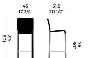
688/A sgabello alto \ barstool
