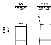
688/AC sgabello alto \ barstool
