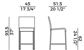
688/SC sgabello basso \ counterstool
